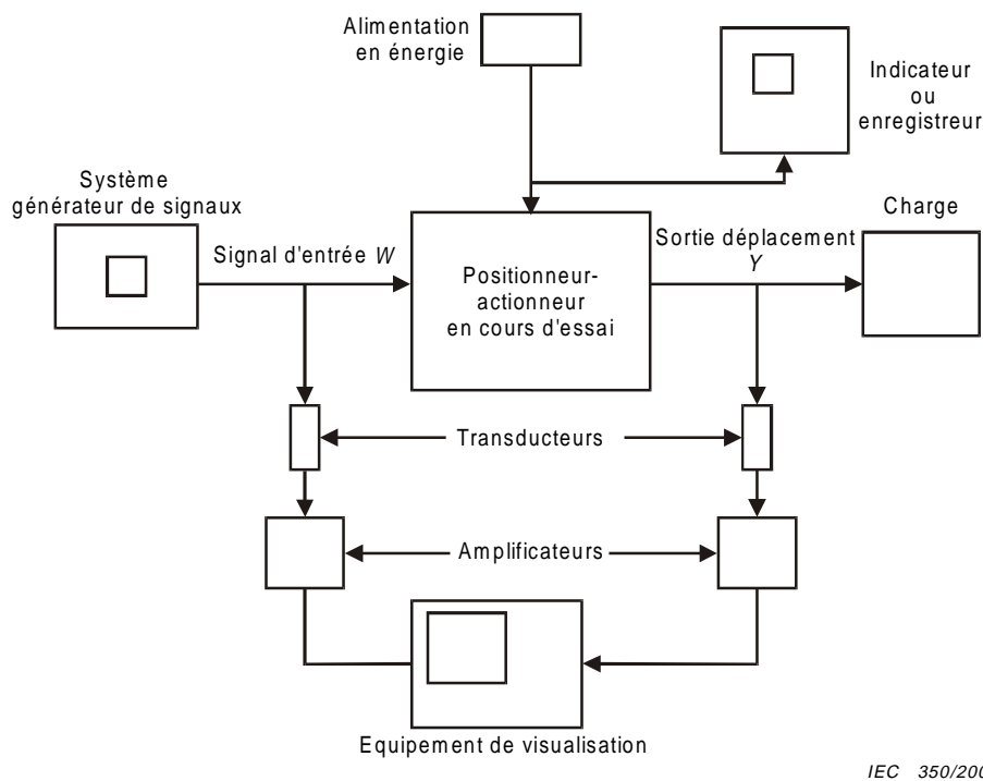
Figure 8 – Disposition d'essai simple pour la mesure de réponse dynamique
