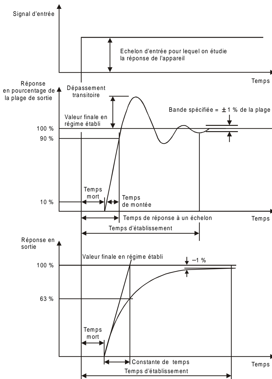
Figure 10 – Deux exemples de réponse à une entrée en échelon
