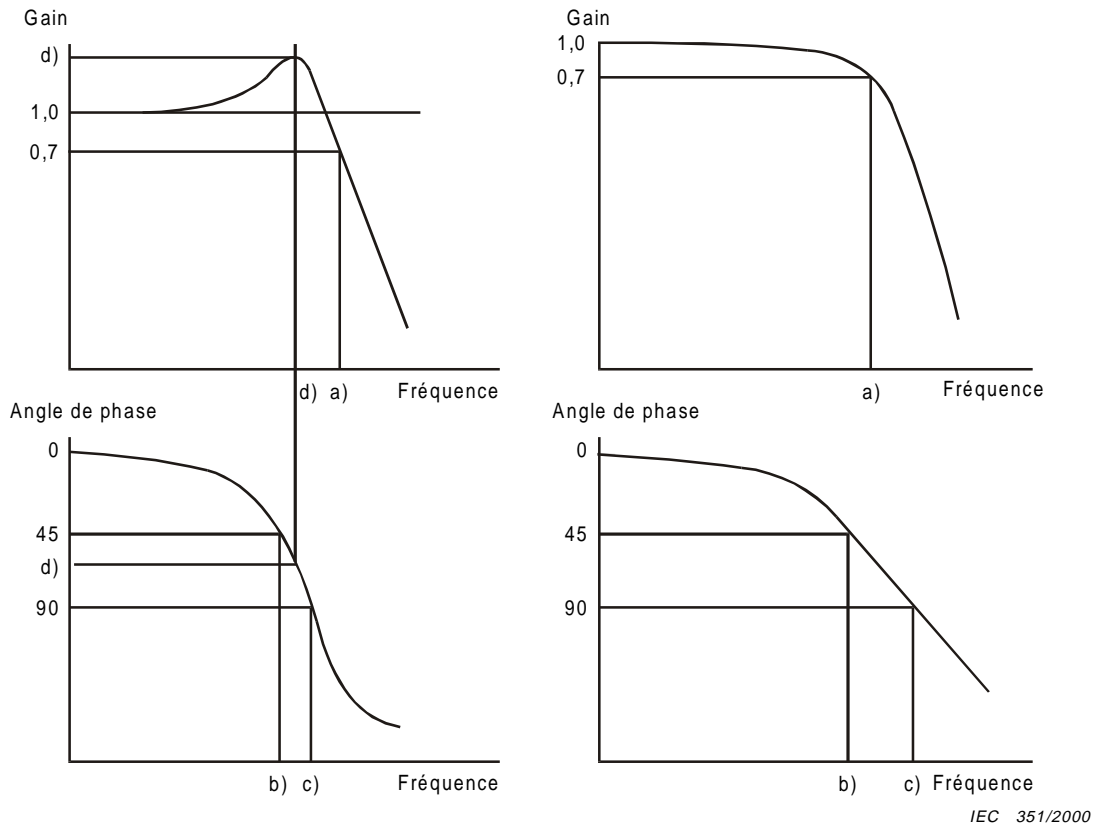
Figure 9 – Deux exemples de réponse harmonique
